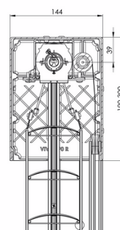
Dwarsdoorsnede van de zichtbare zelfdragende jaloezie
